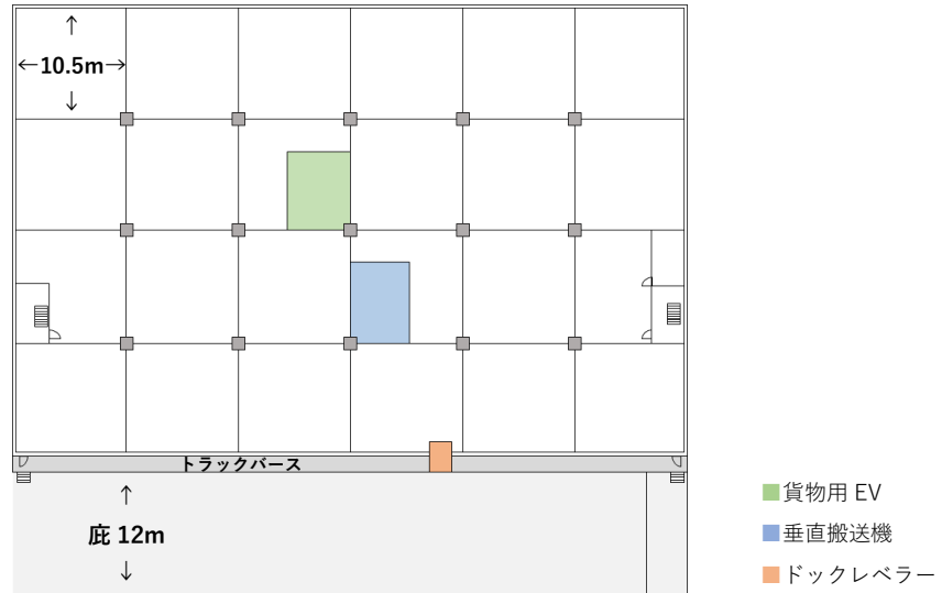
【平面図 (1階)】
