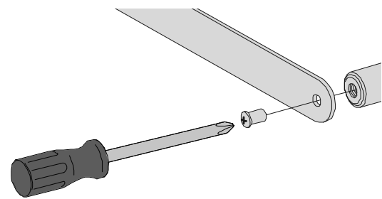
① アングルとハンガーパイプ固定
